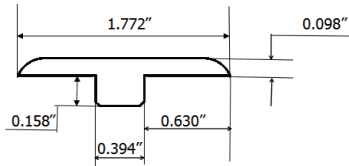
T-molding
